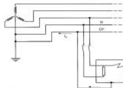
Figura 3. Esquema TN-S.
